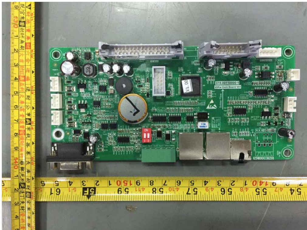
图 16 通讯板
