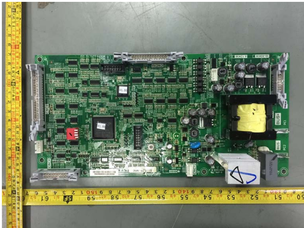
图 12 控制板
