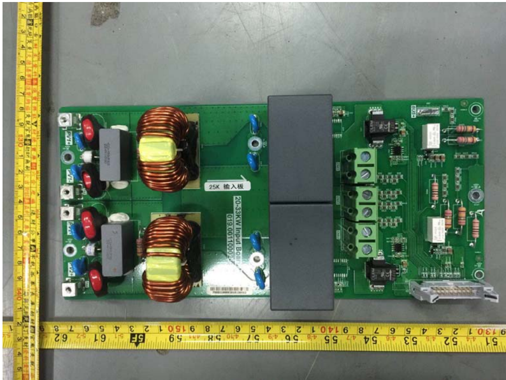
图 15 输入板
