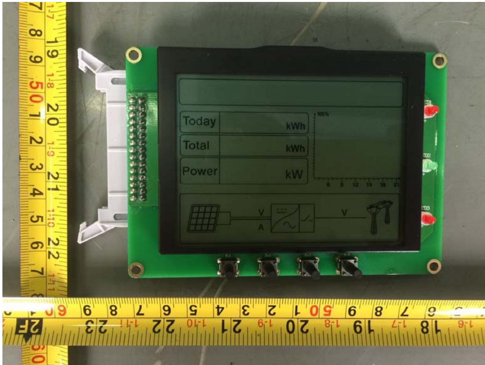
图 11 LCD 板
